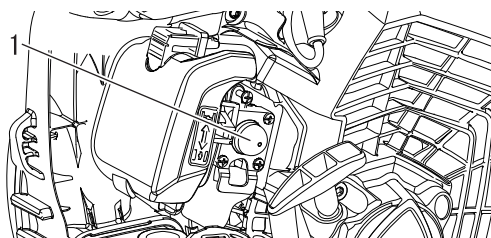
1. Kraftstoffpumpe
