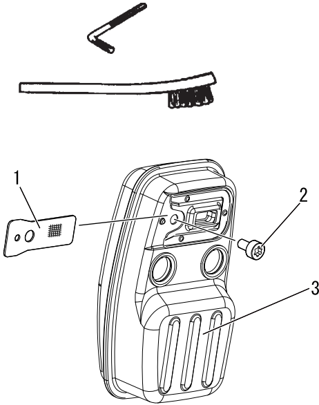
1. Funkenschutzsieb 3. Schalldämpfer
