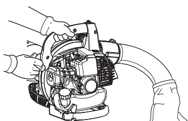
1. Reversierstarter
