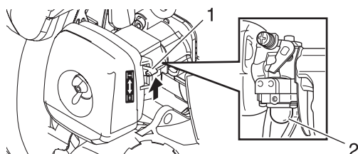
1. Choke 2. Kraftstoffpumpe
